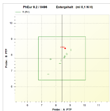
Abb. 2: X-/Y-Diagramm, systematische Abweichung
