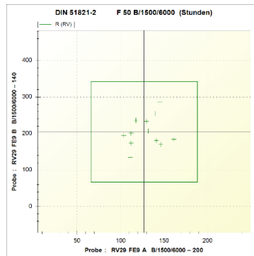
Abb. 1: X-/Y-Diagramm, zufällige Abweichung
